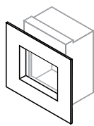
SF4
